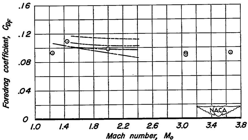
(d) Model No. 14, L—V Haack, \frac{L}{D} = 3 .
