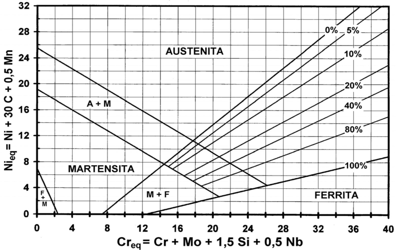
Diagrama de Schaeffler
