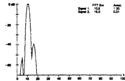
Fig. 73. de la Vallé-Poussin window.
