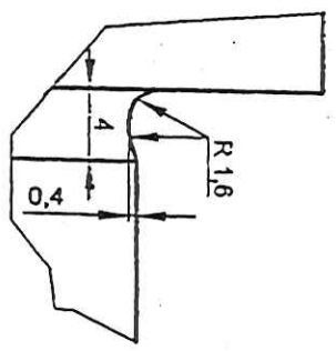
DETALHE B
