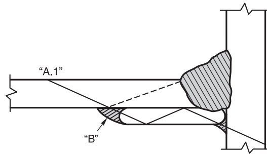
(B) T-JOINTS
