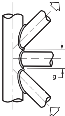
① K(T-K)
