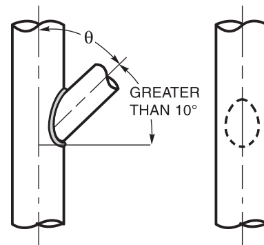
(D) Y-CONNECTION
