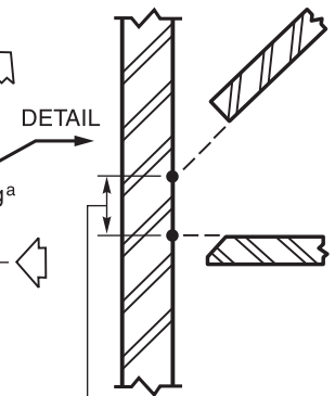
(D) Y-CONNECTION
