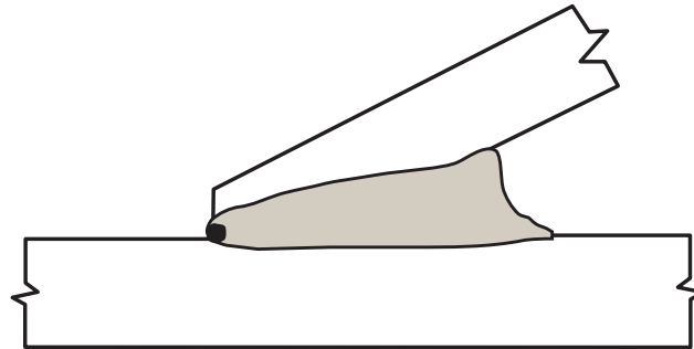
(E) T-, Y-, K-GROOVE WELDS
