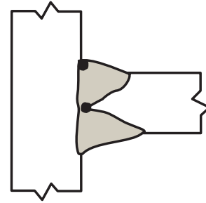
(D) GROOVE T-WELD
