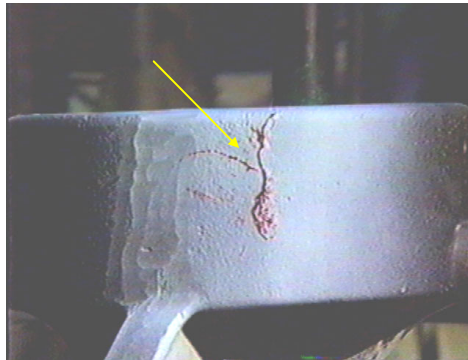
Resultado do ensaio por líquidos penetrantes de uma peça fundida.
