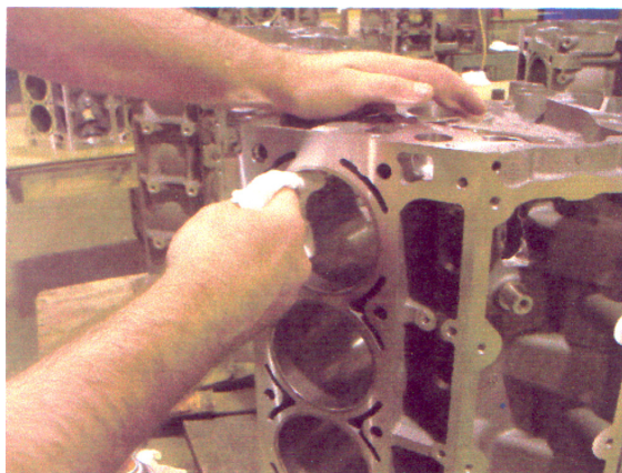
Limpeza com pano após o tempo de penetração de 15 minutos
