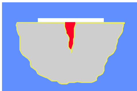
Aplicação do revelador e observação da indicação
