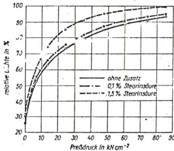
Bild 4.34. Der Einfluß von Stearinsäurezusätzen auf die Verdichtbarkeit von Elektrolytpulver (nach [4.35])
