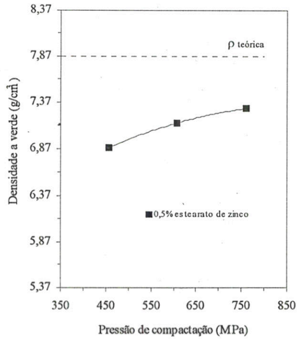
Figura 3.3- Curva de compactabilidade do pó de ferro Ancorsteel 1000C.
