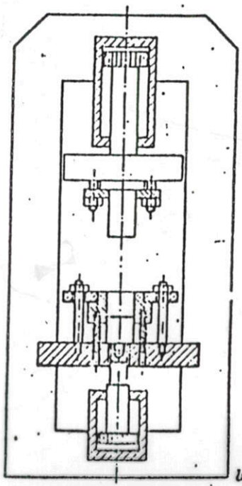
Bild 5.13. Prinzip einer Exzentri.-presse (a) und einer hydraulischen Presse (b) (nach P. Krall)
