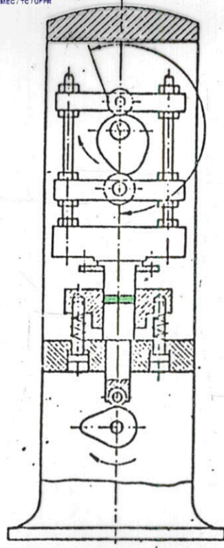
Bild 5.13. Prinzip einer Exzentri.-presse (a) und einer hydraulischen Presse (b) (nach P. Krall)
