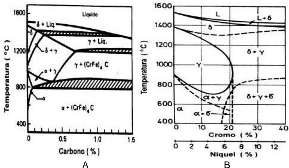
Figura 1- (a) Diagrama de fase pseudobinário Fe-C com 12%Cr; (Welding Handbook, v. 4, 1998); b) Diagrama de equilíbrio pseudo-binário Fe-Cr-Ni (Folkhard, 1988).
