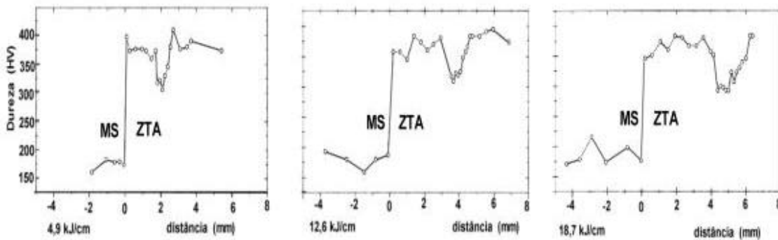
Figura 4- Perfis de dureza obtidos junto à seção transversal dos cordões depositados com diferentes níveis de energia sobre o aço CA-6NM temperado, utilizando eletrodo revestido AWS E NiCrFe-2.
