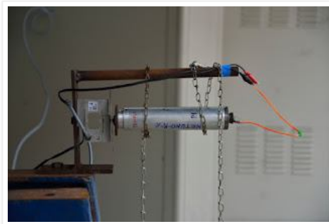
Motor-foguete Netuno-R-Beta preparado para teste estático na UFPR em 4 Nov 2018. Foto: Thiago L. Quevedo
