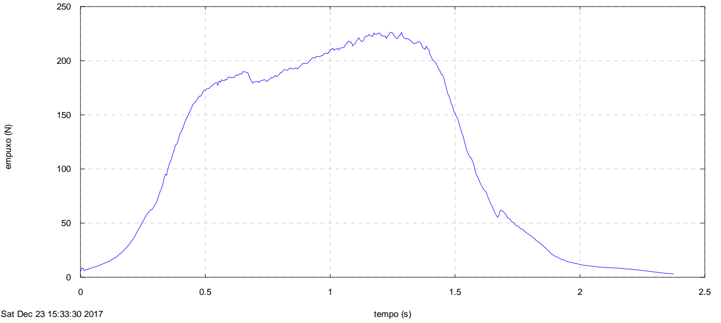
Motor Urano, teste 19, TE 10 Dez 2017, Curva Empuxo 2.1
