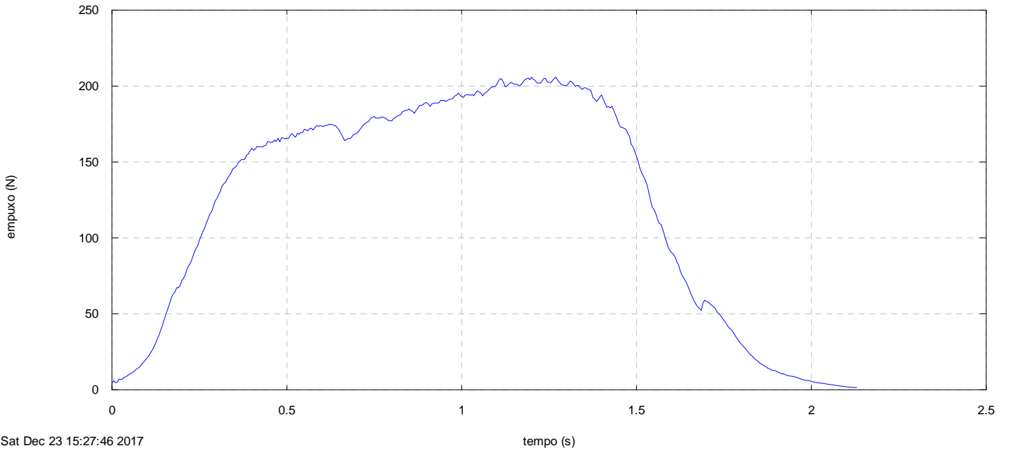
Motor Urano, teste 18, TE 10 Dez 2017, Curva Empuxo 2.1
