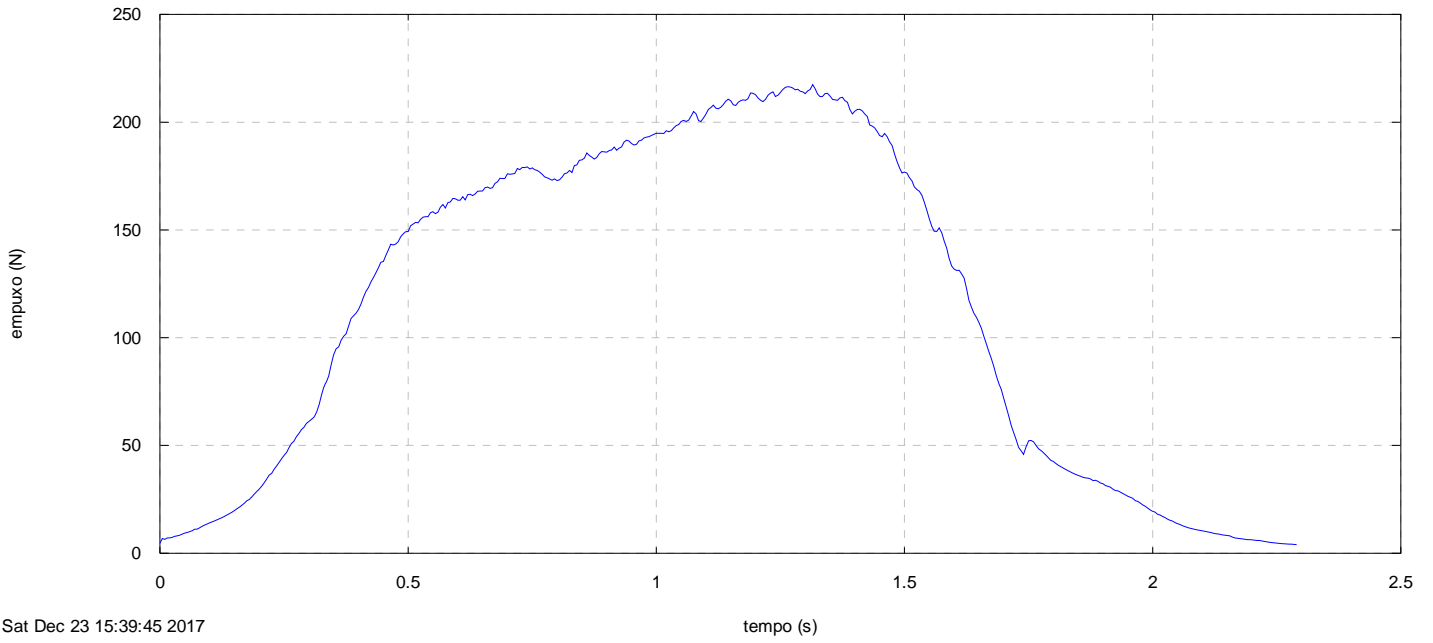
Motor Urano, teste 20, TE 10 Dez 2017, Curva Empuxo 2.1
