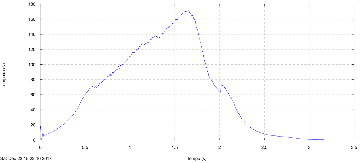
Motor Urano, teste 17, TE 10 Dez 2017, Curva Empuxo 2.1
