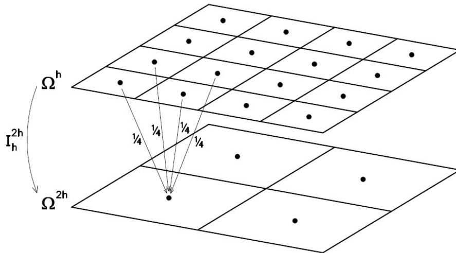
FIGURA 12 – OPERADOR DE RESTRIÇÃO COM PONDERAÇÃO EM 2D.
