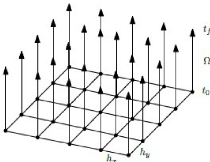
FIGURA 25 – ATUALIZAÇÃO DAS INCÓGNITAS COM VARREDURA WAVEFORM RELAXATION 2D .
