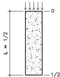
FIGURA 27 – MODELO DO PROBLEMA DA POROELASTICIDADE UNIDIMENSIONAL.
