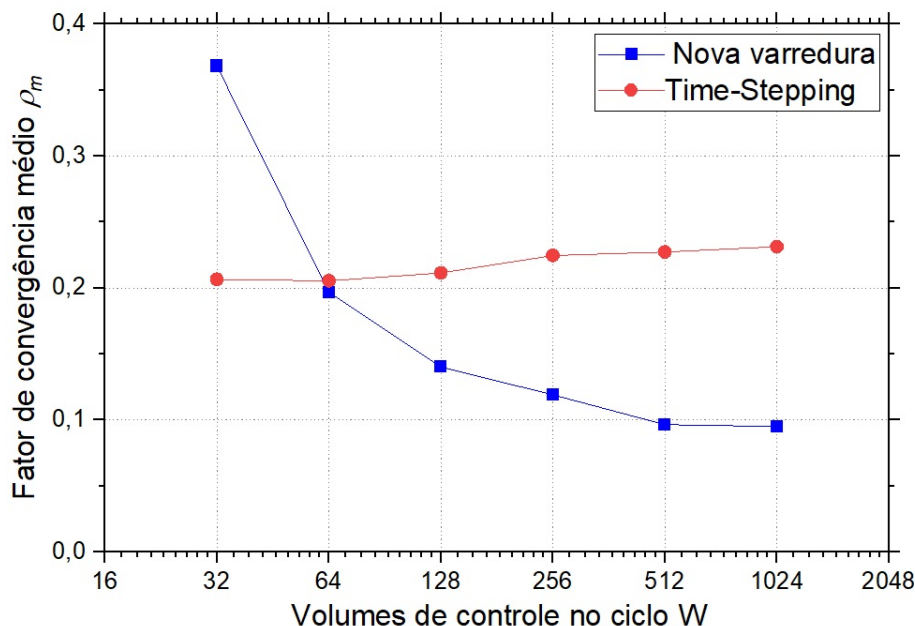
FIGURA 41 – FATOR DE CONVERGÊNCIA COM A VARREDURAS TIME-STEPPING E A NOVA VARREDURA PARA O CASO 3.
