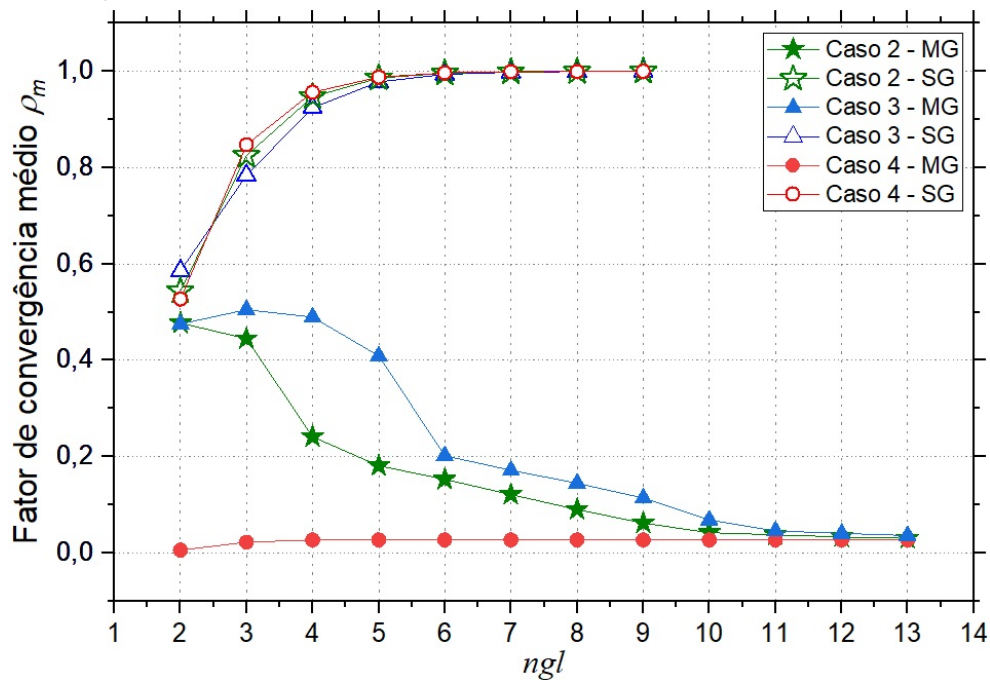
FIGURA 43 – COMPARATIVO DE \rho_m ENTRE SINGLEGRID E MULTIGRID PARA OS CASOS 2, 3 e 4.
