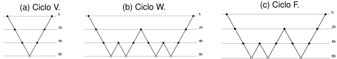
FIGURA 15 – ESTRUTURA DOS CICLOS V, W E F COM QUATRO NÍVEIS DE MALHA.
