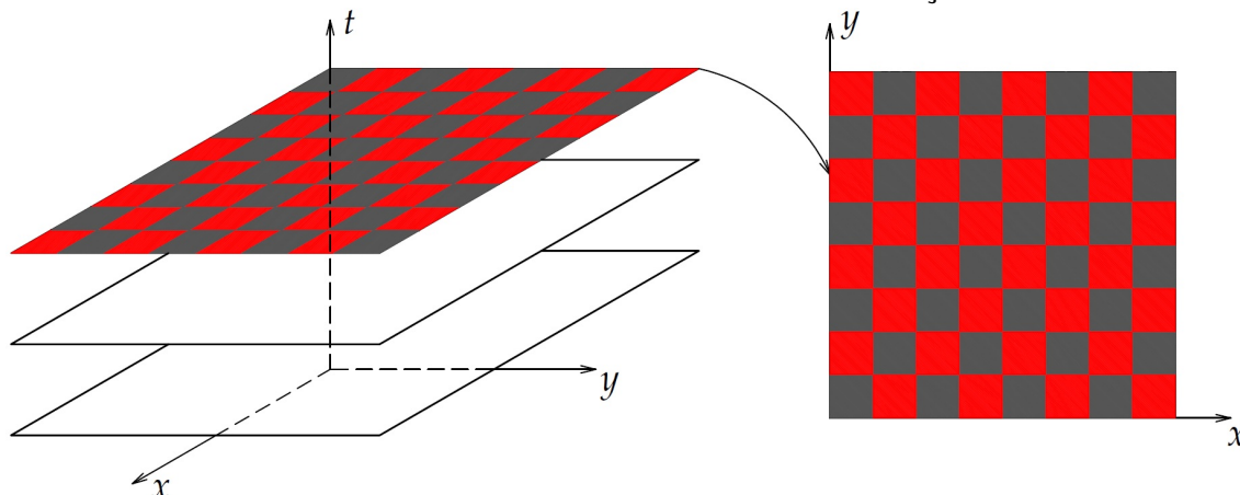
FIGURA 35 – ESQUEMA NOVA VARREDURA ESPAÇO-TEMPO
