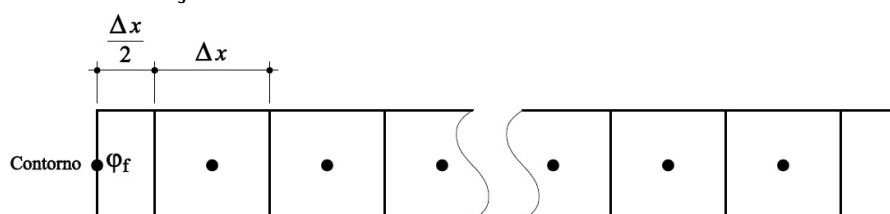
FIGURA 29 – CONDIÇÃO DE CONTORNO USANDO MEIO VOLUME NA FRONTEIRA
