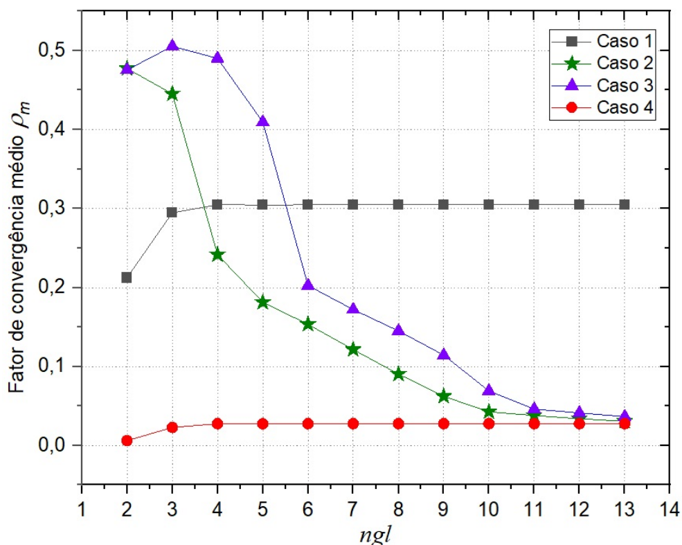
FIGURA 44 – COMPARATIVO \rho_m PARA O MULTIGRID DEFINIDO PARA OS 4 CASOS ESTUDADOS.
