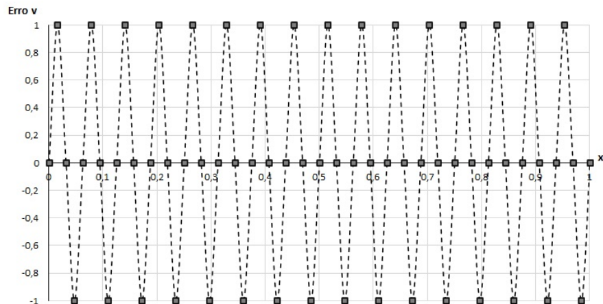
FIGURA 6 – MODO OSCILATÓRIO k = 32 PARA UMA MALHA COM \mathcal{N} = 64 VOLUMES.
