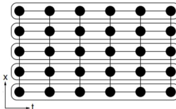
FIGURA 24 – ATUALIZAÇÃO DAS INCÓGNITAS COM VARREDURA WAVEFORM RELAXATION 1D .
