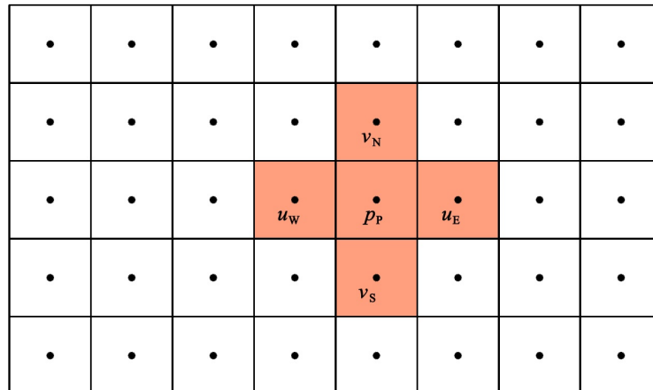
FIGURA 17 – SUAVIZADOR VANKA NO PROBLEMA DA POROELASTICIDADE 2D.
