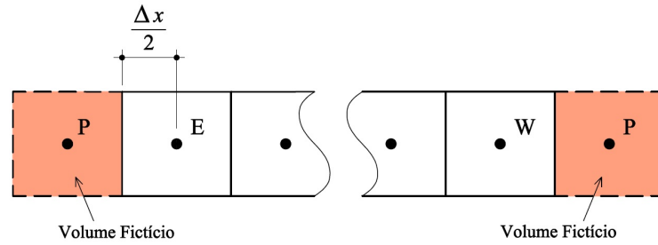
FIGURA 30 – CONDIÇÃO DE CONTORNO USANDO VOLUMES FICTÍCIOS NA FRONTEIRA.
