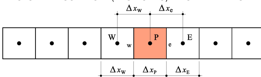
FIGURA 28 – VOLUME DE CONTROLE (DESTACADO) EM UMA MALHA UNIDIMENSIONAL.
