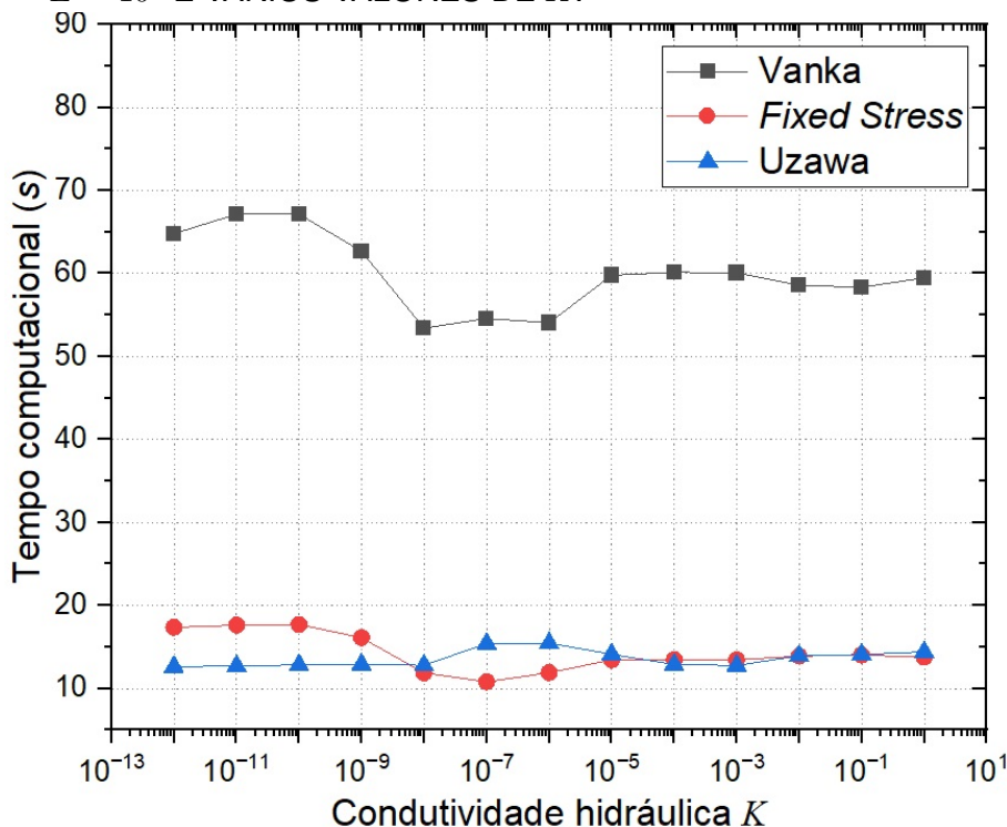
FIGURA 38 – TEMPO COMPUTACIONAL EM FUNÇÃO DO VALOR DE K COM N = 1024 E E = 10^4 E VÁRIOS VALORES DE K .
