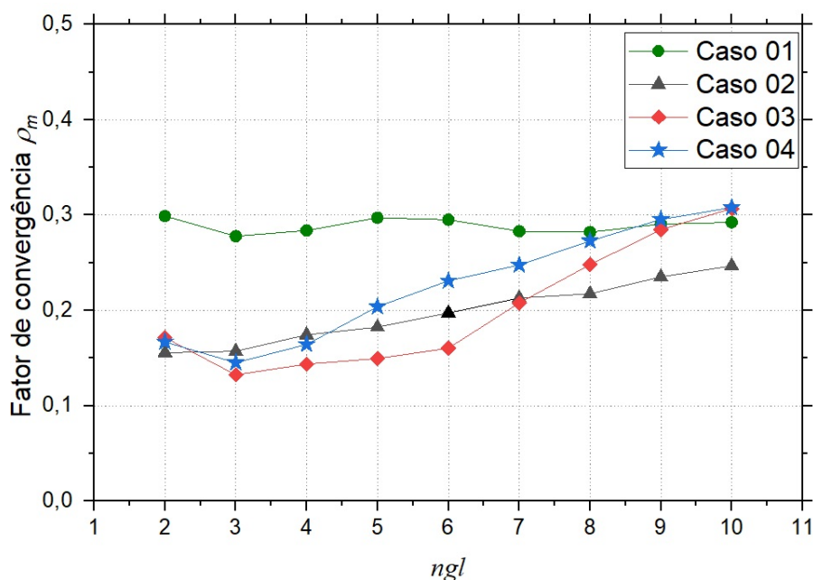
FIGURA 39 – MÉTODO UZAWA
