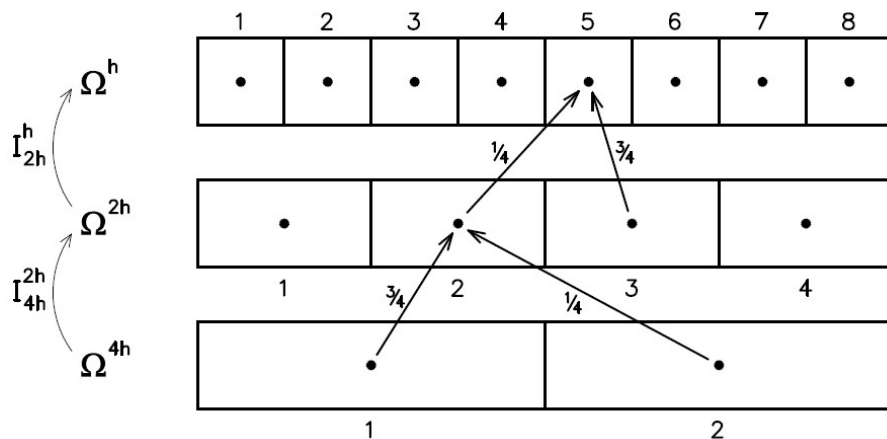
FIGURA 13 – OPERADOR DE PROLONGAÇÃO EM 1D.
