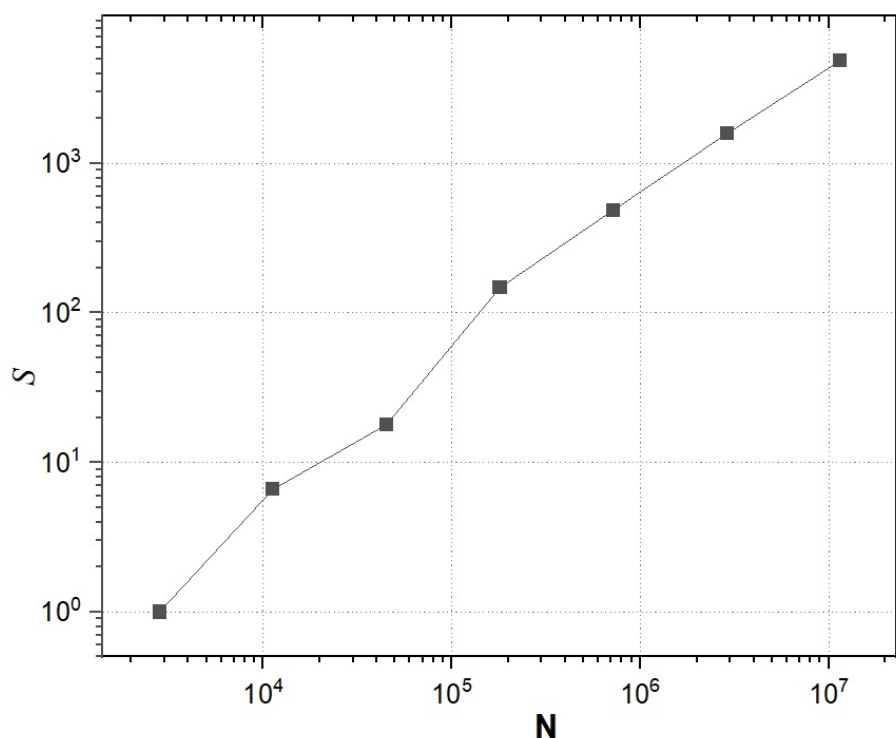
FIGURA 46 – SPEED-UP PARA O CASO 4.
