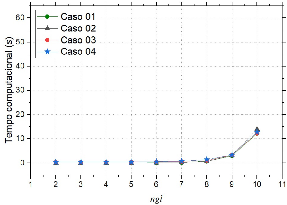
FIGURA 51 – TEMPO COMPUTACIONAL PARA O MÉTODO FIXED-STRESS
