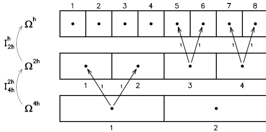
FIGURA 14 – OPERADOR DE PROLONGAÇÃO EM 1D.
