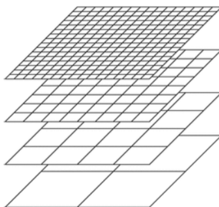
FIGURA 9 – MÚLTIPLAS MALHAS COM RAZÃO DE ENGROSSAMENTO 2 NO ESPAÇO 2D.
