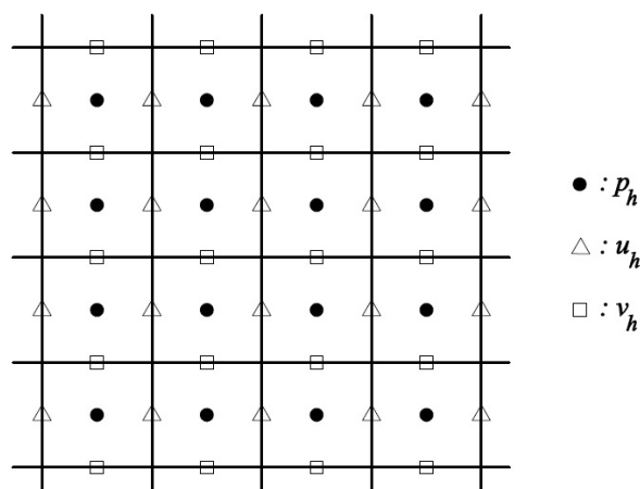
FIGURA 34 – MALHA UNIFORME 2D COM VARIÁVEIS DESENCONTRADAS.
