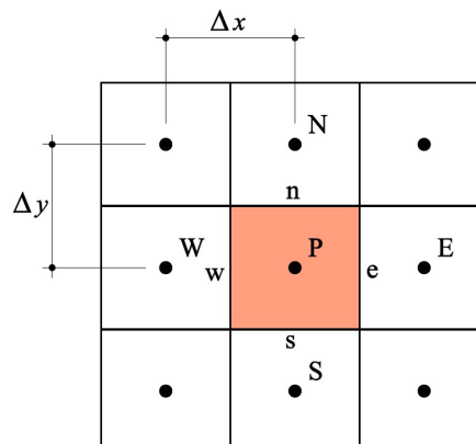
FIGURA 32 – DESCRIÇÃO DO VOLUME DE CONTROLE EM UMA MALHA 2D.
