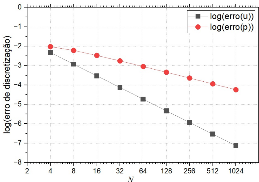
FIGURA 36 – ERRO DE DISCRETIZAÇÃO UTILIZANDO FIXED-STRESS COM E = 10^4 E K = 1 .
