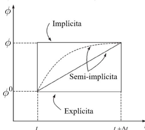
FIGURA 20 – FUNÇÕES DE INTERPOLAÇÃO DA VARIÁVEL TEMPORAL.
