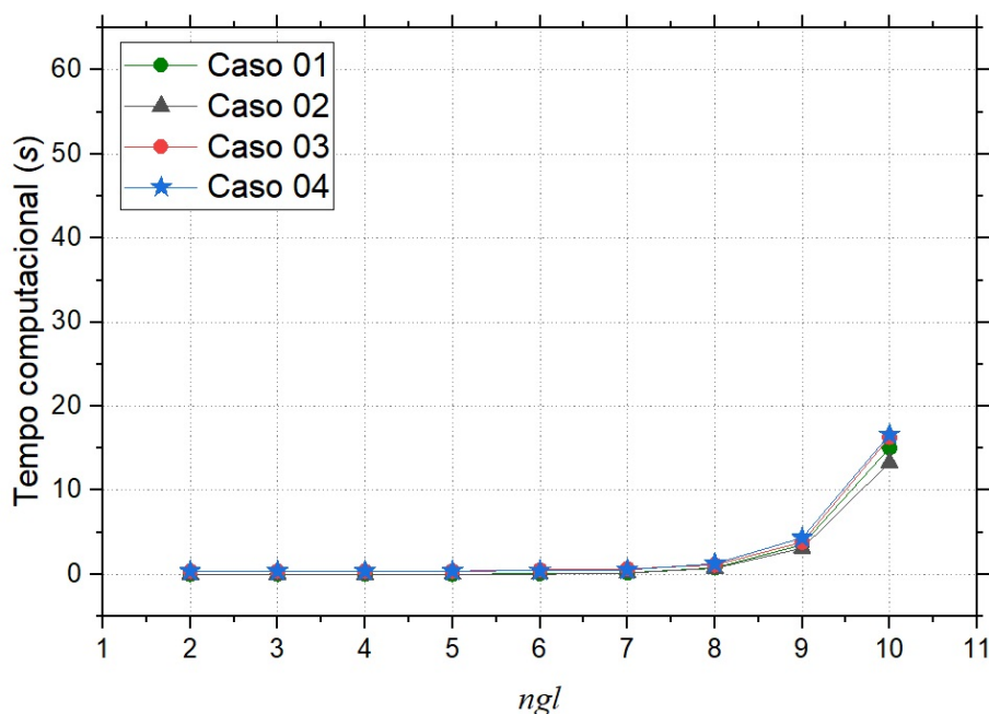
FIGURA 40 – TEMPO COMPUTACIONAL PARA O MÉTODO UZAWA
