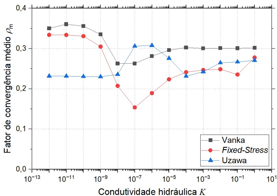
FIGURA 37 – FATOR DE CONVERGÊNCIA MÉDIO \rho_m EM FUNÇÃO DO VALOR DE K PARA A MALHA COM N = 1024 VOLUMES E E = 10^4 E VÁRIOS VALORES DE K .
