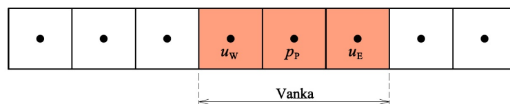
FIGURA 16 – SUAVIZADOR VANKA NO PROBLEMA 1D.
