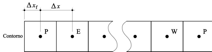
FIGURA 31 – CONDIÇÃO DE CONTORNO USANDO BALANÇO DE VOLUMES NA FRONTEIRA.
