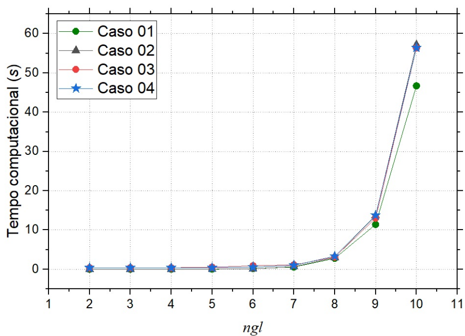
FIGURA 49 – TEMPO COMPUTACIONAL PARA O MÉTODO VANKA
