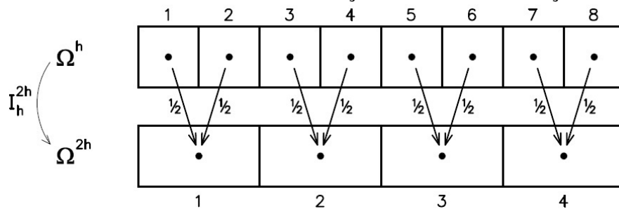
FIGURA 11 – OPERADOR DE RESTRIÇÃO COM PONDERAÇÃO EM 1D.
