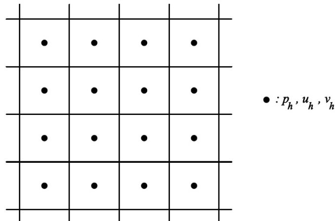
FIGURA 33 – MALHA UNIFORME 2D COM AS VARIÁVEIS COLOCALIZADAS.
