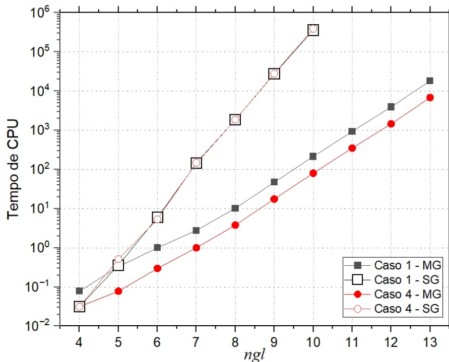
FIGURA 45 – TEMPO DE CPU PARA SG E MG COM O REFINO DAS MALHAS.
