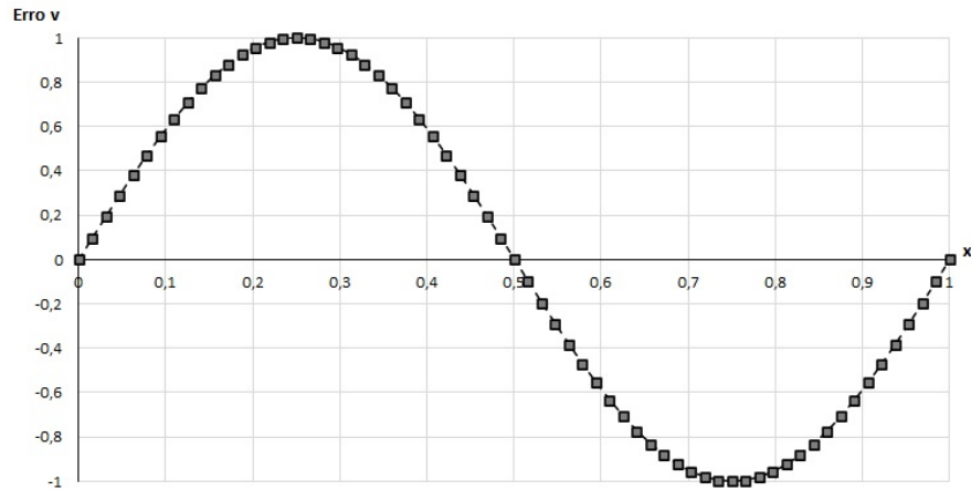
FIGURA 5 – MODO SUAVE k = 2 PARA UMA MALHA COM \mathcal{N} = 64 VOLUMES.
