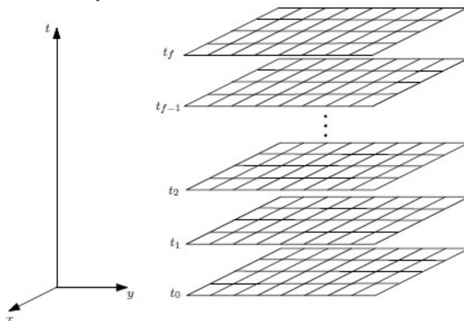
FIGURA 23 – ATUALIZAÇÃO DAS INCÓGNITAS COM A VARREDURA TIME-STEPPING 2D.
