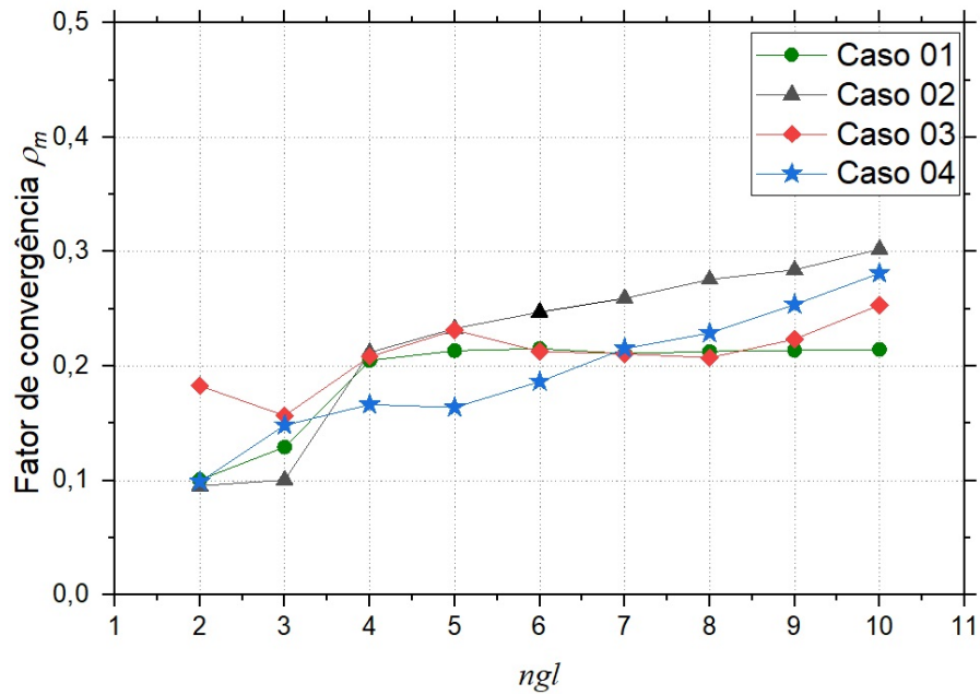
FIGURA 48 – FATOR DE CONVERGÊNCIA PARA O MÉTODO VANKA
