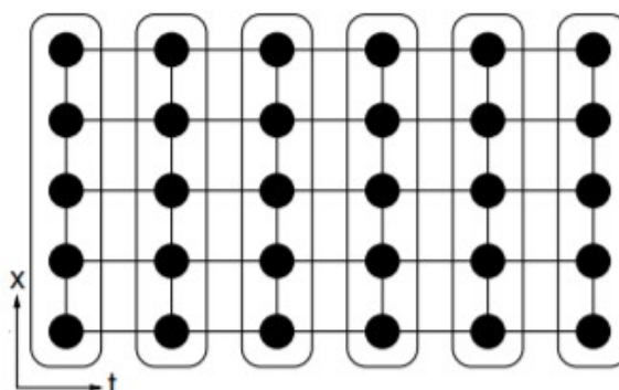
FIGURA 22 – ATUALIZAÇÃO DAS INCÓGNITAS COM A VARREDURA TIME-STEPPING 1D
