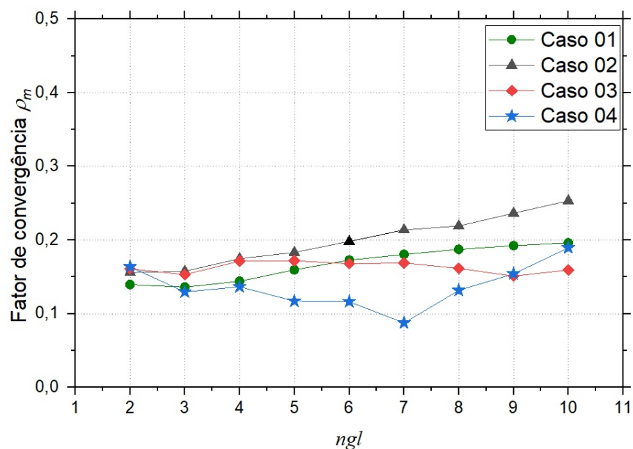
FIGURA 50 – FATOR DE CONVERGÊNCIA PARA O MÉTODO FIXED-STRESS
