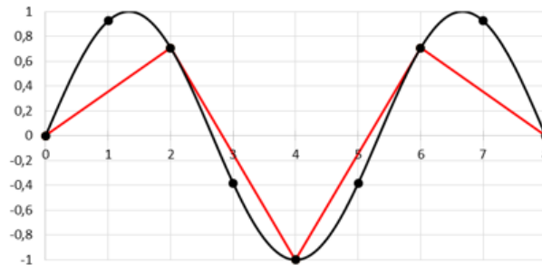
FIGURA 10 – MODOS SUAVES (CONSIDERANDO 9 PONTOS) E OSCILATÓRIOS (CONSIDERANDO 5 PONTOS).
