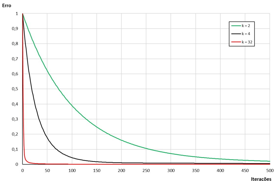
FIGURA 7 – NORMA INFINITO DO ERRO VERSUS NÚMERO DE ITERAÇÕES PARA ESTIMATIVAS INICIAIS COM MODOS k = 2 , k = 4 E k = 32 , USANDO GAUSS-SEIDEL LEXICOGRÁFICO PARA A EQUAÇÃO DE POISSON.
