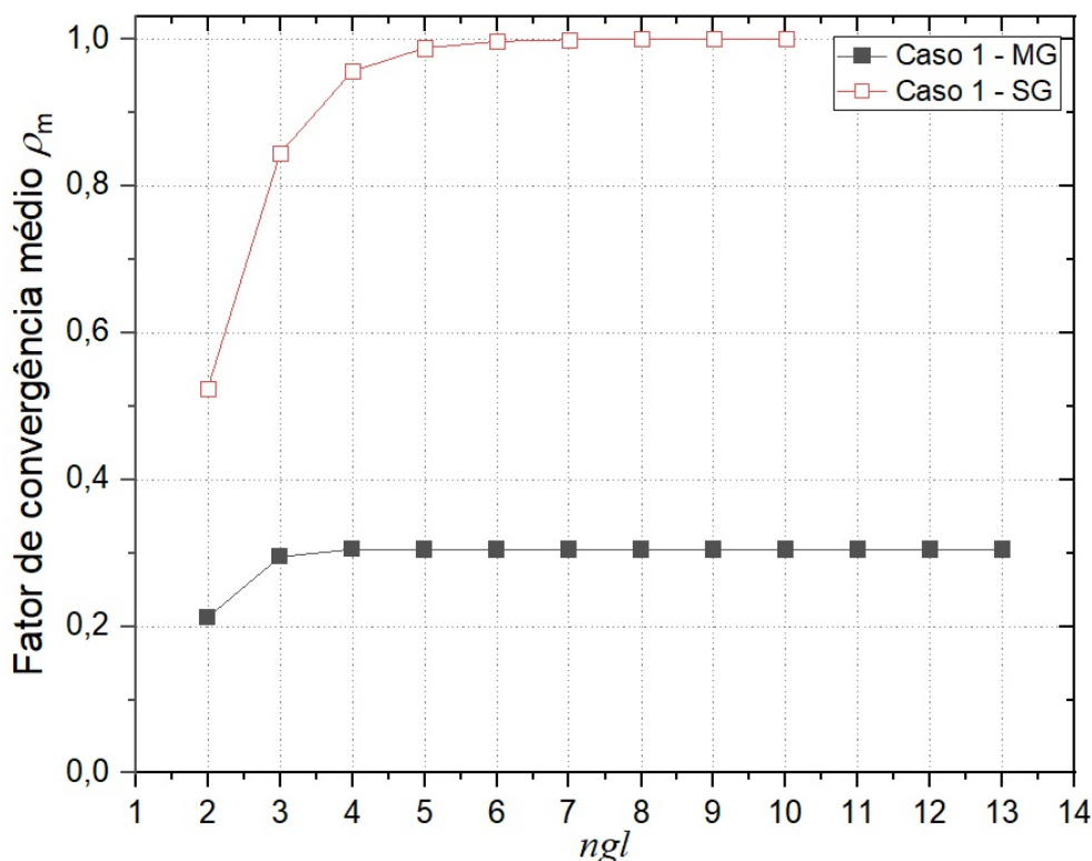
FIGURA 42 – COMPARATIVO DE \rho_m ENTRE SINGLEGRID E MULTIGRID PARA O CASO 1.
